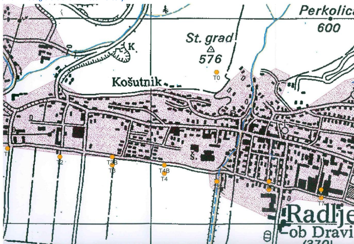
Slika 24: Geografska shema mest vzorčenja
